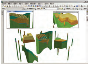
地质体建模，实现了对钻孔、岩层和断层等信息的可视化以及剖切面分析，辅助研究地质结构
