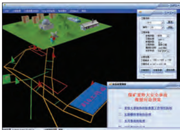
矿山瓦斯动态监测预警系统，为煤矿通风安全管理提供了集成的数据环境和自动化的管理平台
